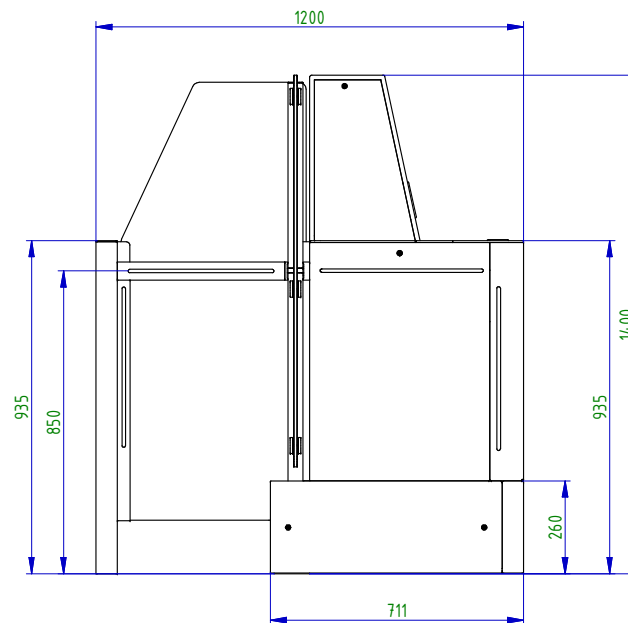
A-A ( 1 : 15 )
