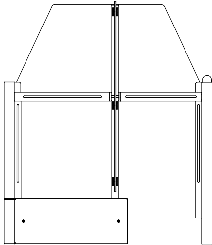
B-B ( 1 : 15 )
